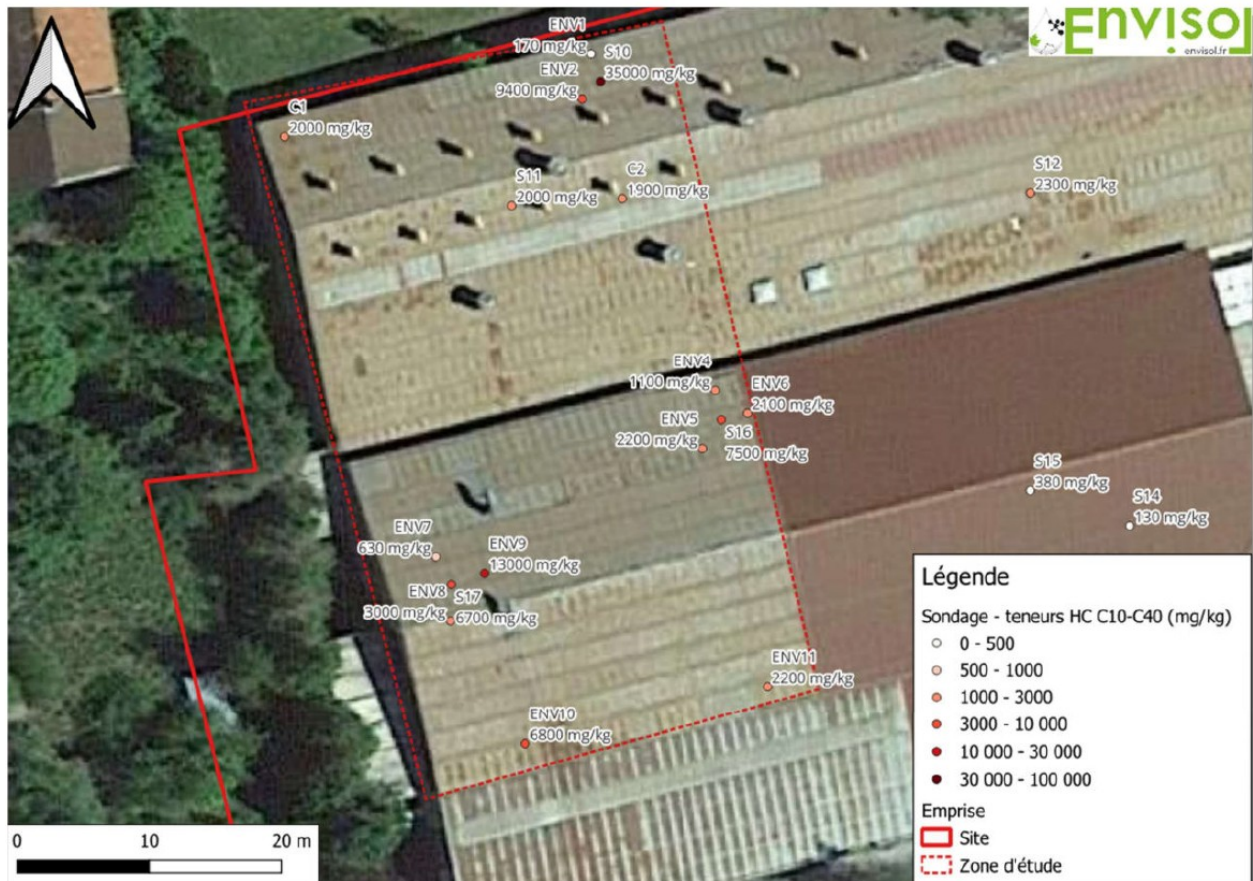
Figure 16 : Présentation de la synthèse des résultats en hydrocarbures – sols (sondage S de 2015 et ENV de 2023)
